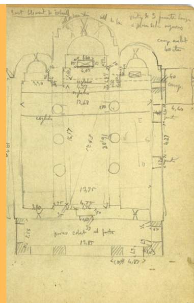
Planta de St.Climent de Taüll. Quadern de notes de J.Puig i Cadafalch.1907
