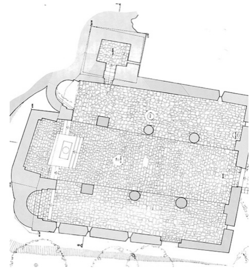
Planta basilical actual de l'església de St Joan de Boí.
