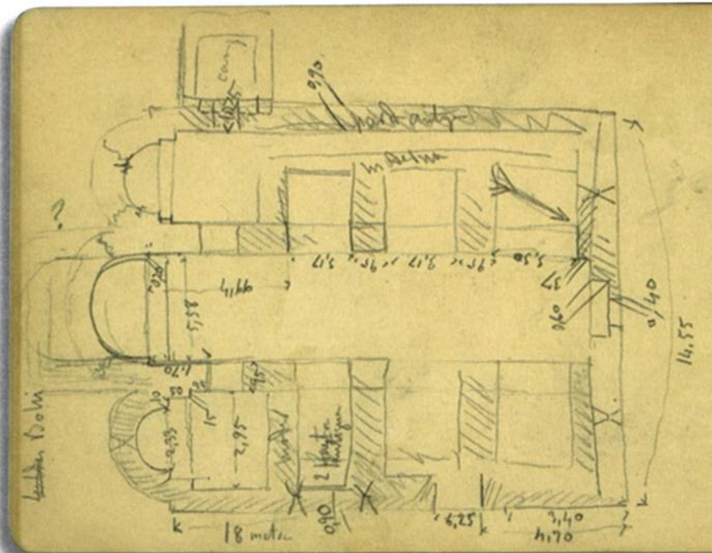
Planta de l'església de Sant Joan de Boí. Quadern de notes de J.Puig i Cadafalch. 1907.
